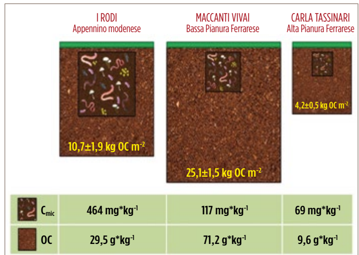
FIG. 3 CARICA MICROBICA E CARBONIO ORGANICO NEI SUOLI
