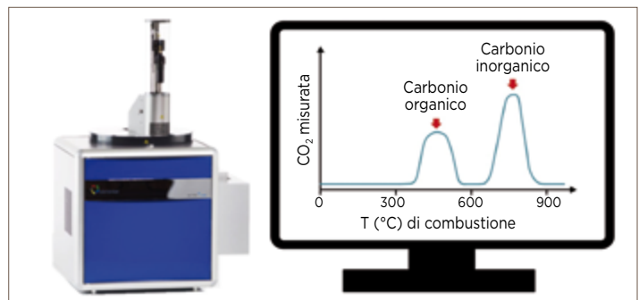
FIG. 2 QUANTIFICAZIONE DEL CARBONIO
