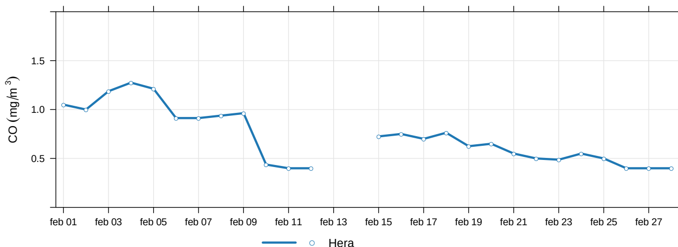
Figura 2: Massimi giornalieri della media di 8 ore di monossido di carbonio.
