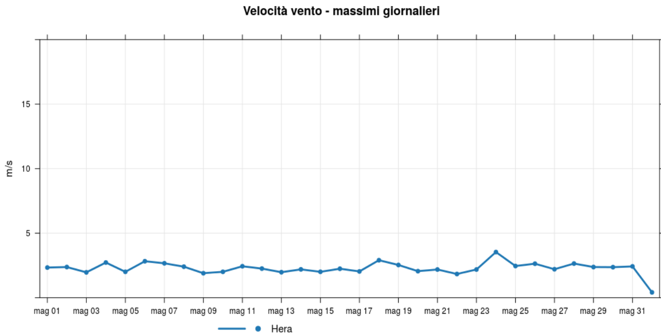
Figura 8: Velocità del vento – Massimi giornalieri
