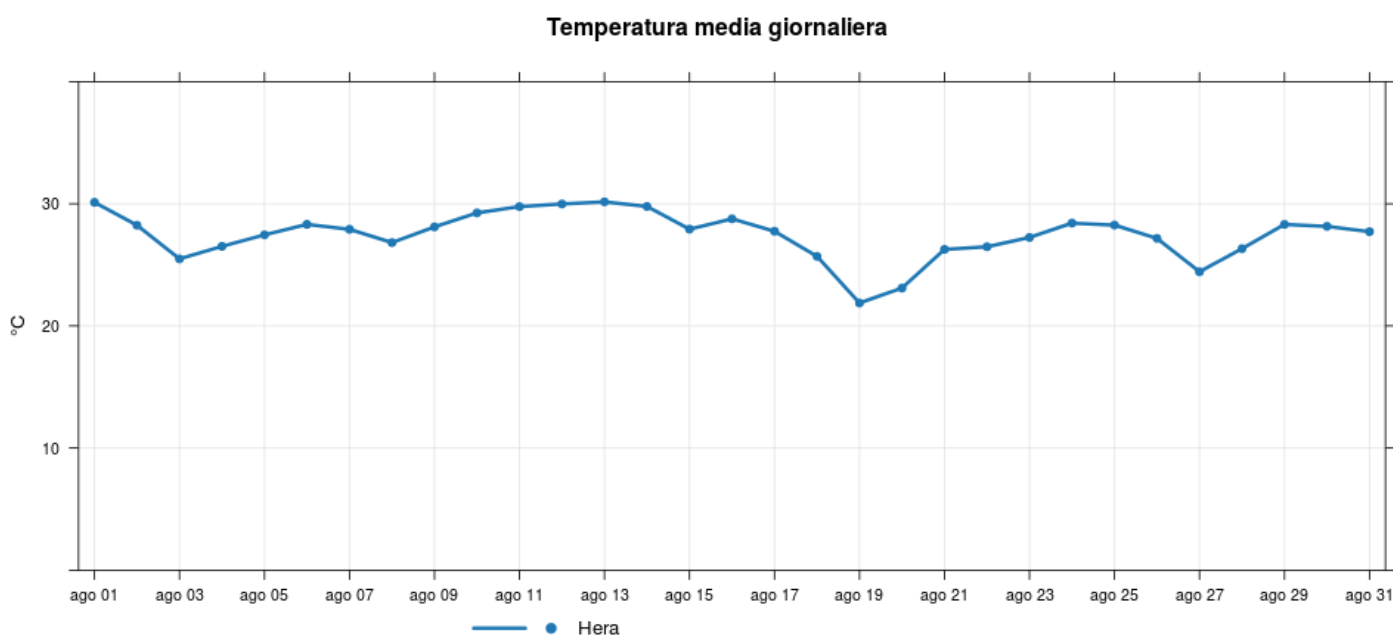
Figura 9: Temperatura media giornaliera
