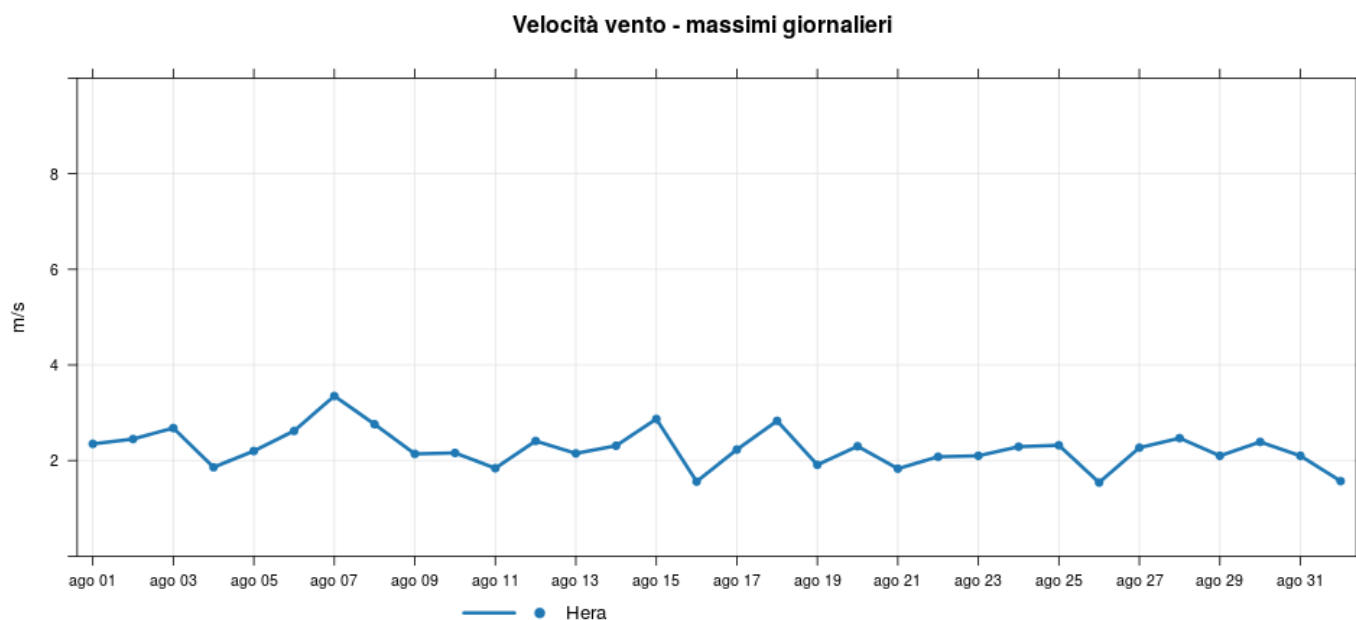
Figura 8: Velocità del vento – Massimi giornalieri
