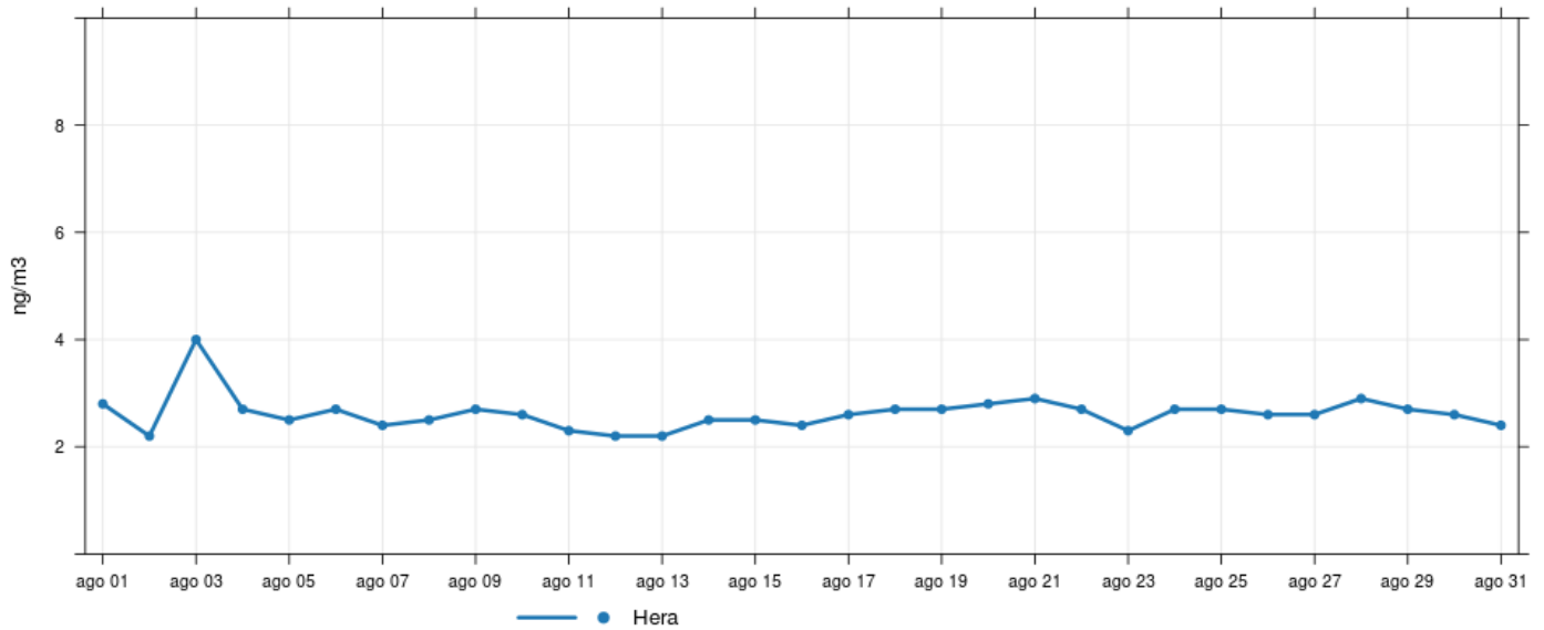
Mercurio - Massimi giornalieri
