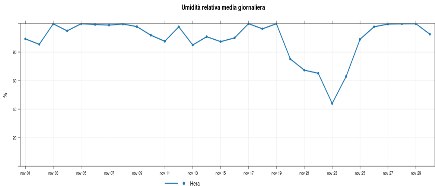
Figura 10:Umidità relativa media giornaliera
