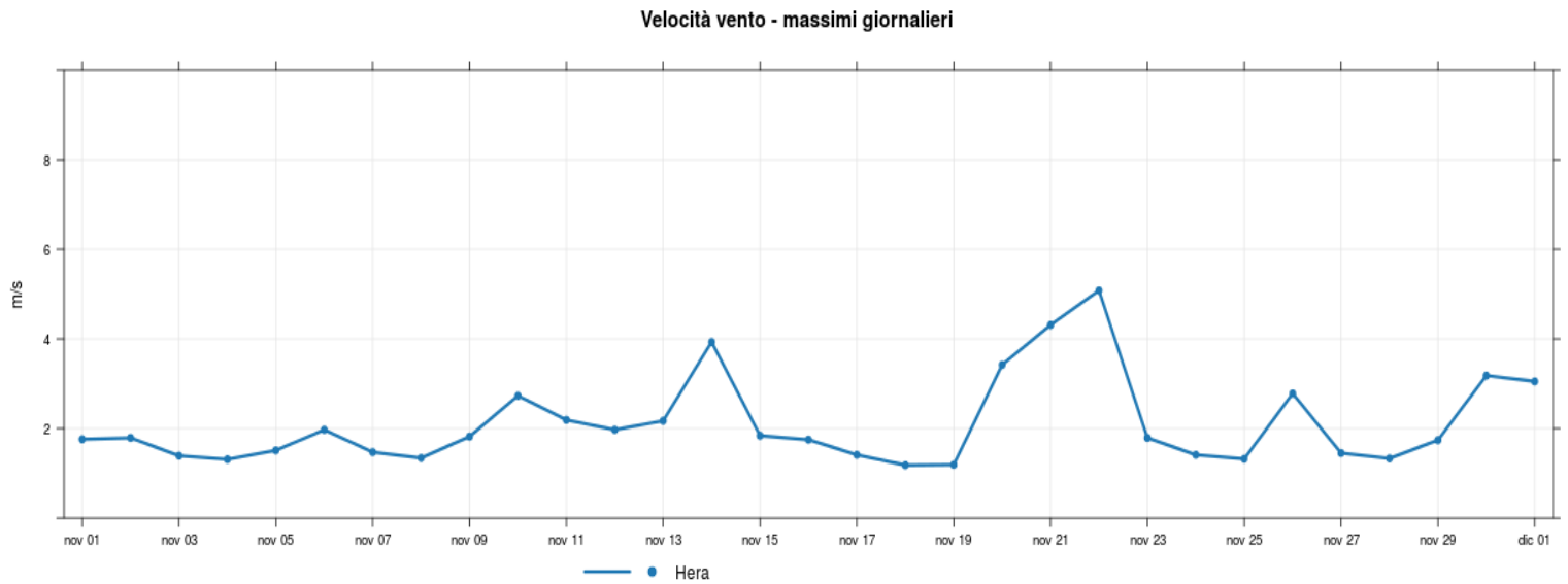
Figura 8: Velocità del vento – Massimi giornalieri
