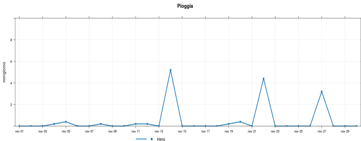
Figura 11:Pioggia cumulata nell'arco delle 24 ore
