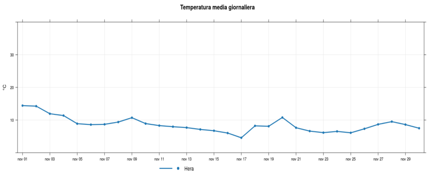
Figura 9: Temperatura media giornaliera
