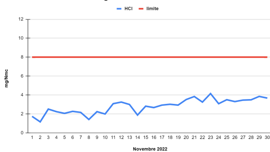
Valore medio giornaliero ACIDO CLORIDRICO
