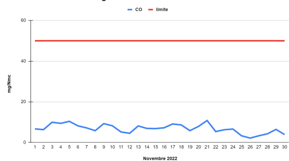
Valore medio giornaliero MONOSSIDO DI CARBONIO
