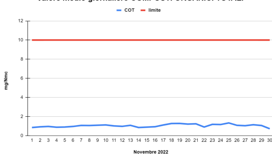
Valore medio giornaliero COMPOSTI ORGANICI TOTALI
