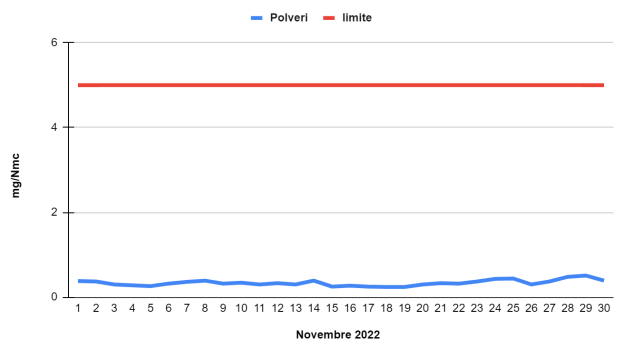
Valore medio giornaliero POLVERI
