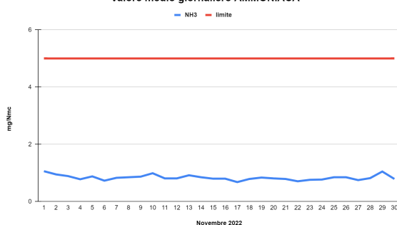
Valore medio giornaliero AMMONIACA
