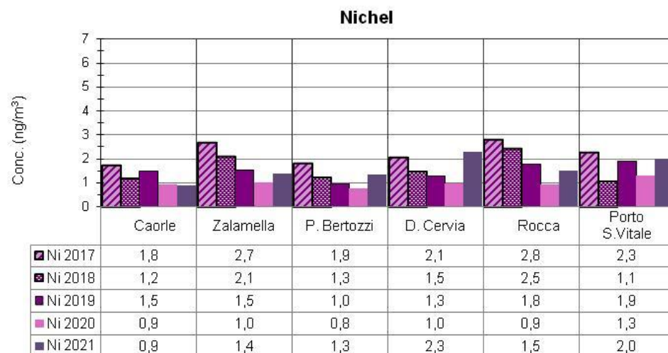
Figura 4.37 – Andamento medie annuali di alcuni metalli nel particolato PM10
