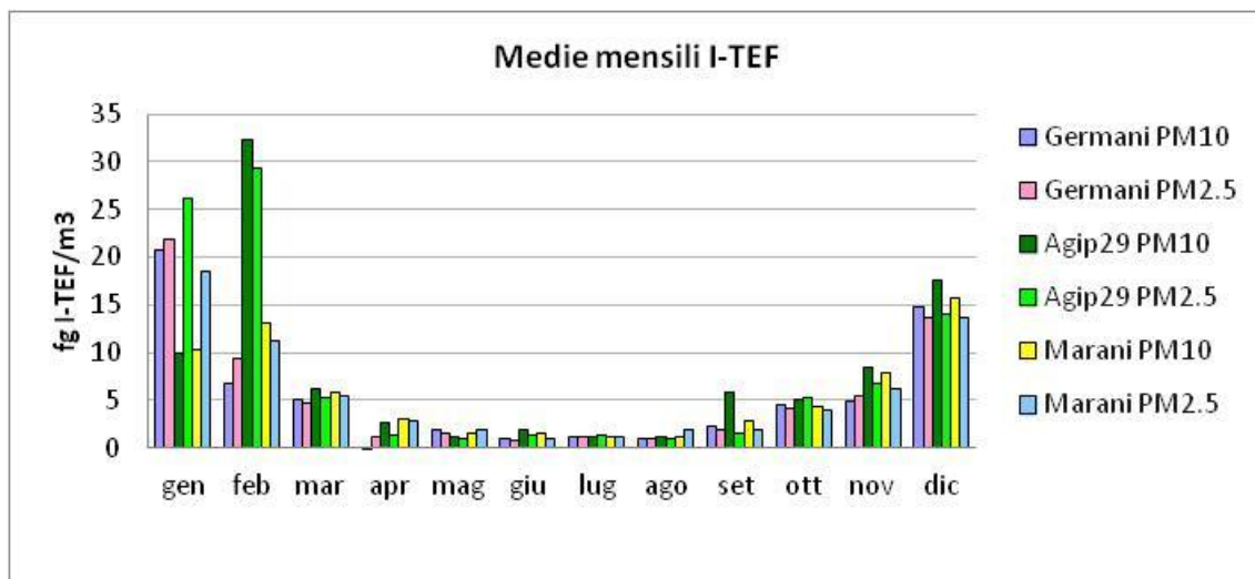
Figura 4.41 – Tossicità equivalente per sommatoria di PCDD, PCDF, PCB - medie mensili 2021
