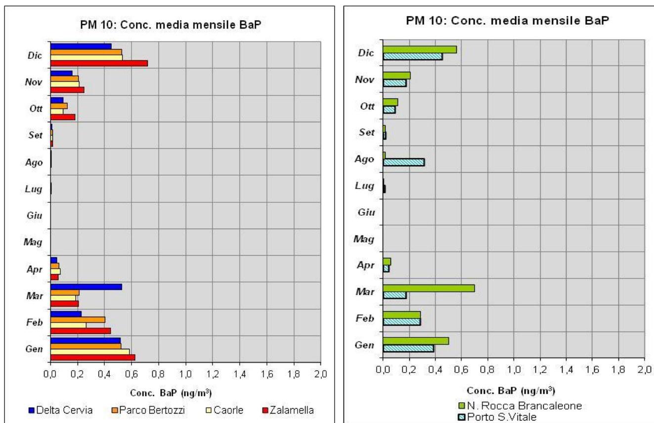
Figura 4.26 – Andamento temporale delle concentrazioni medie mensili di BaP nel PM10 nel 2021 - Stazioni urbane e di fondo (a sinistra) e in stazioni locali industriali (a destra)
