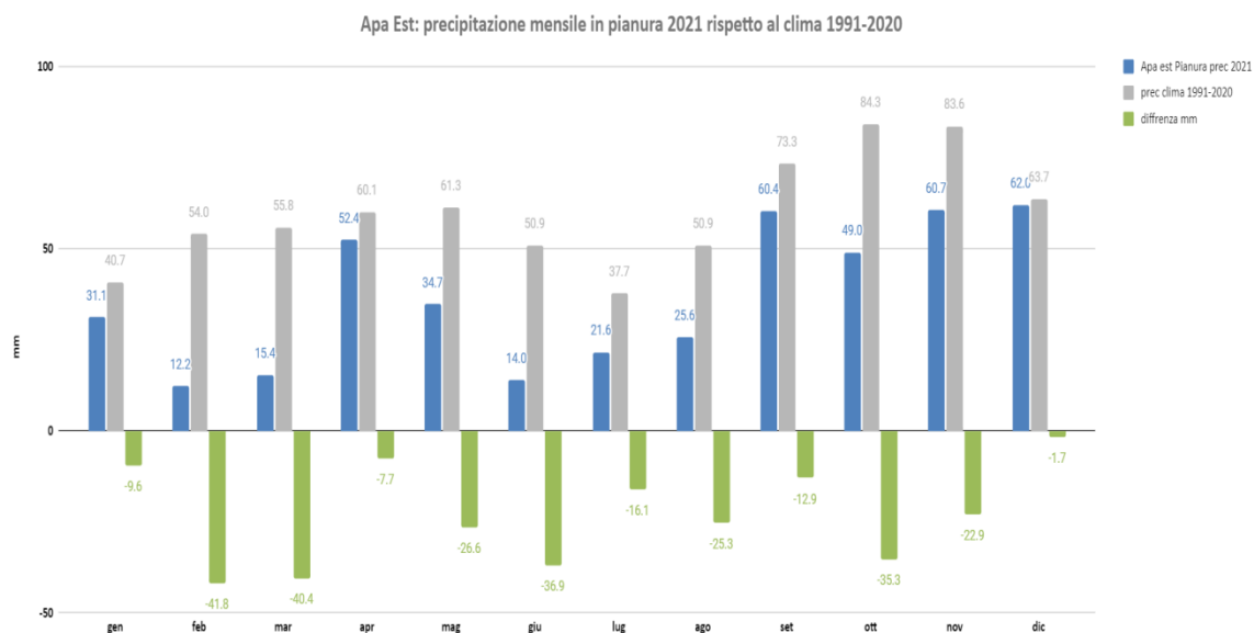
Figura 3.4a: Precipitazioni medie mensili, valori climatici mensili (1991-2020) e anomalie mensili mediate sulle aree di pianura delle tre provincie.
