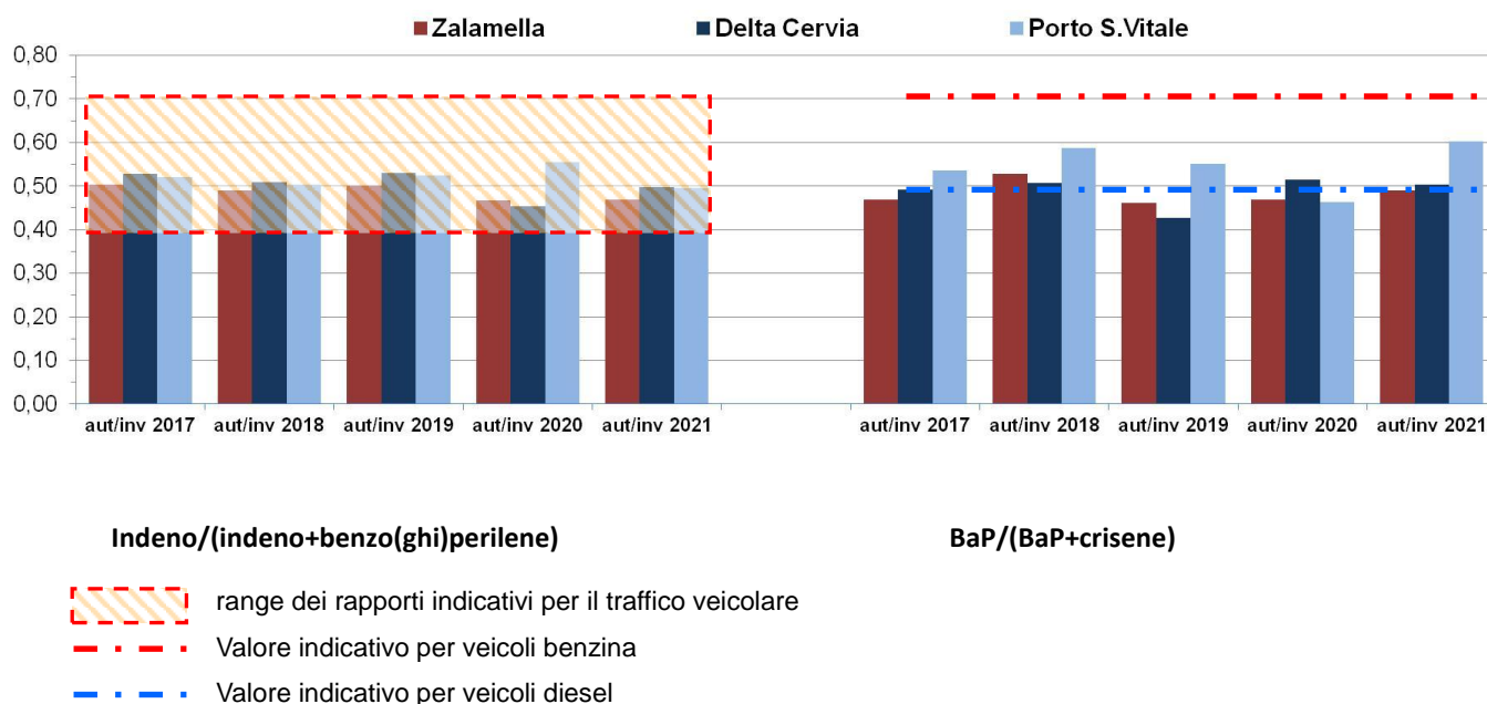
Figura 4.31 – Rapporti diagnostici, mesi invernali e autunnali 2017 – 2021
