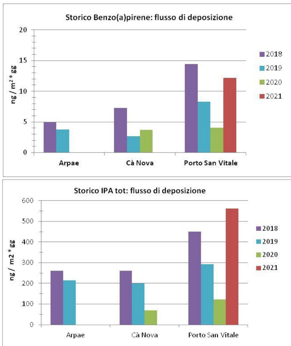
Figura 4.4: Trend medie annuali per Benzo(a)pirene e IPA totali
