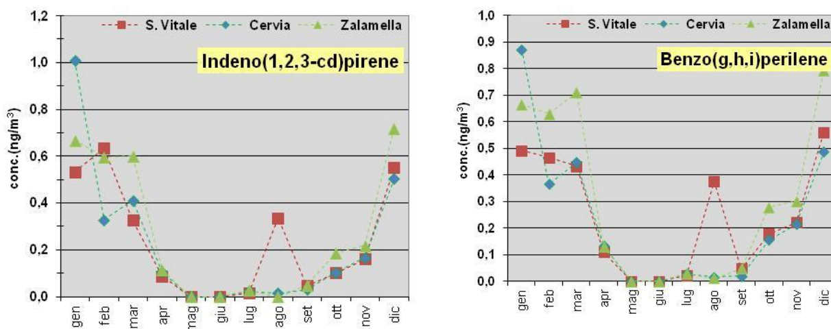
Figura 4.30 – Medie mensili degli IPA considerati nei rapporti diagnostici 2021
