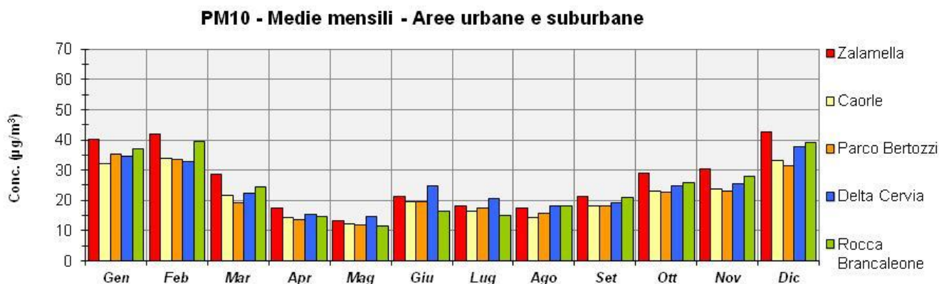
Figura 4.20 – PM10 medie mensili Area Urbana e Sub Urbana – Stazioni RRQA + Stazione Locale di Rocca Brancaleone (Ind/Urb) anno 2021
