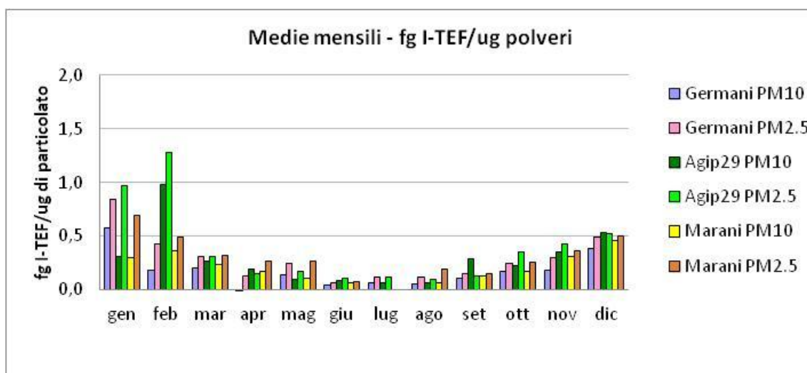
Figura 4.42 – Rapporto fra tossicità equivalente per sommatoria di PCDD, PCDF, PCB e particolato raccolto sui filtri - medie mensili 2021
