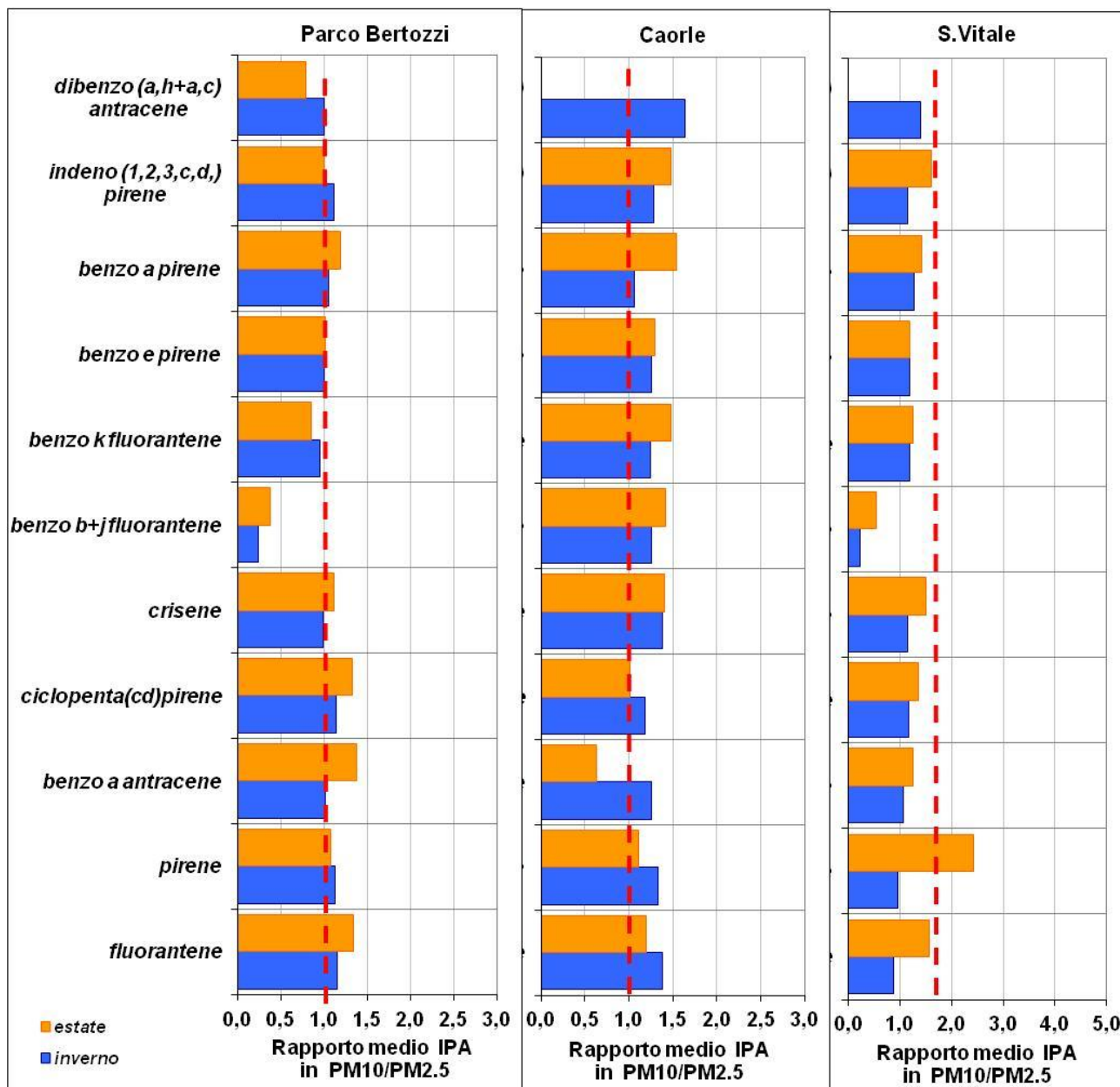
Figura 4.29 – Rapporto “ng IPA per ogni g PM10 / ng IPA per ogni g PM2.5” - Anno 2021
