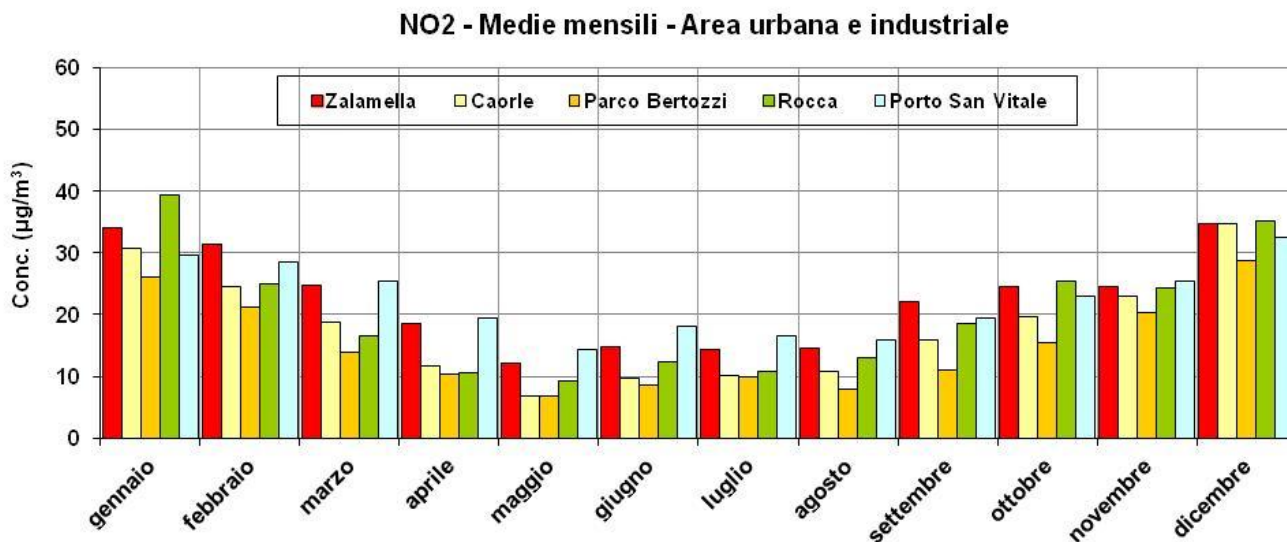
Figura 4.4 Medie Mensili - Area urbana e Industriale
