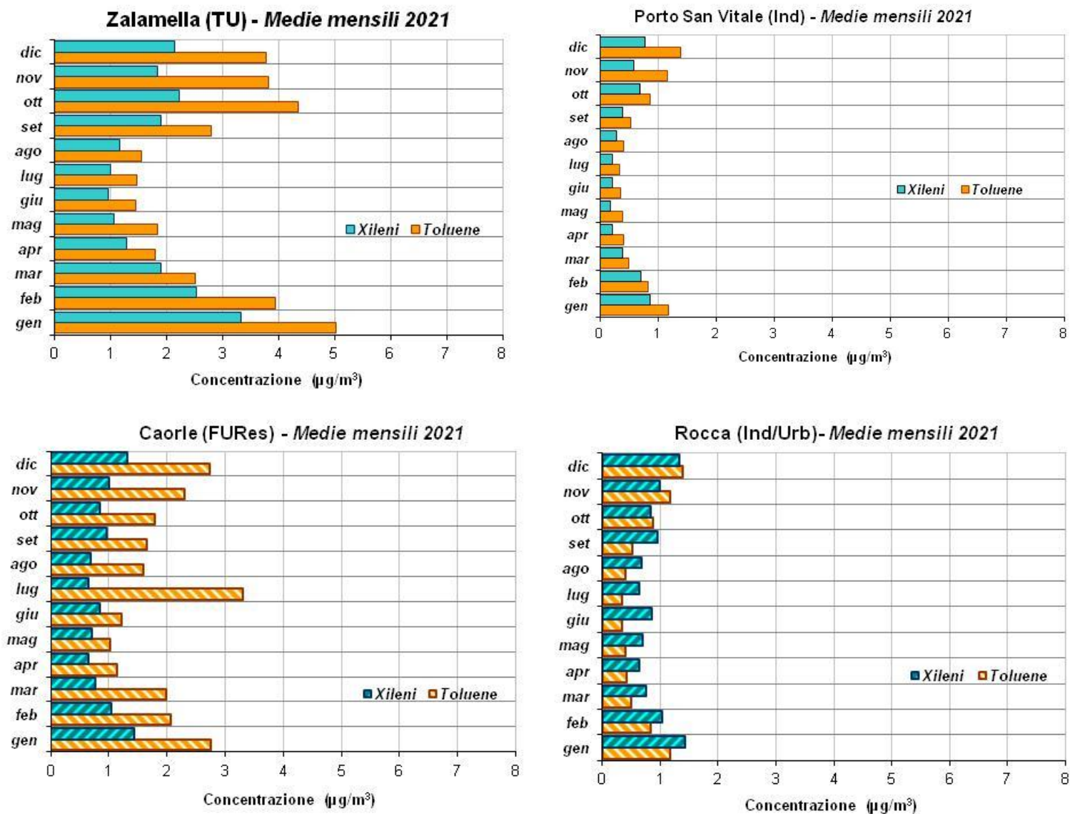
Figura 4.15 – Toluene e Xileni: concentrazioni medie mensili – anno 2021
