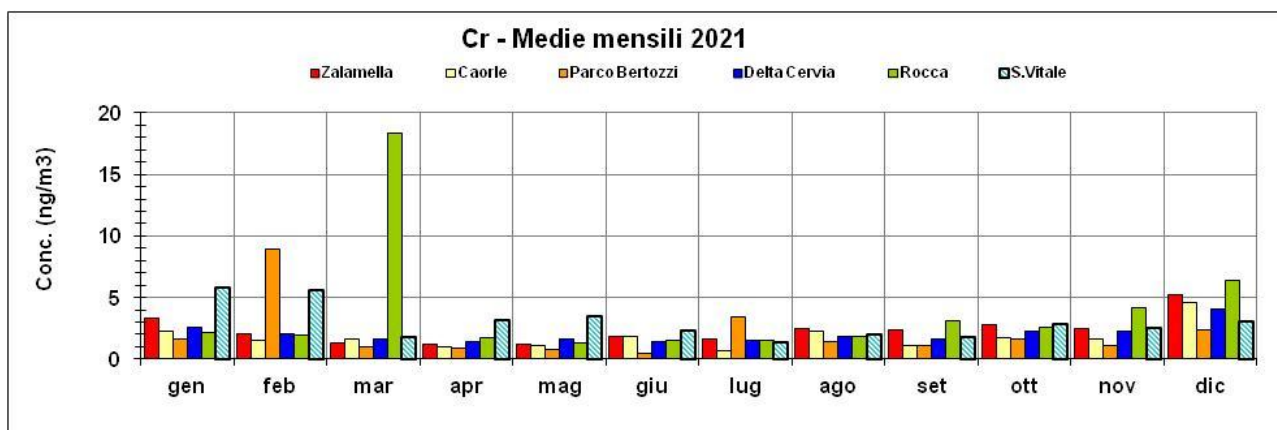
Figura 4.34 (a) – Medie mensili di piombo, cadmio e cromo nel particolato PM10 – Anno 2021
