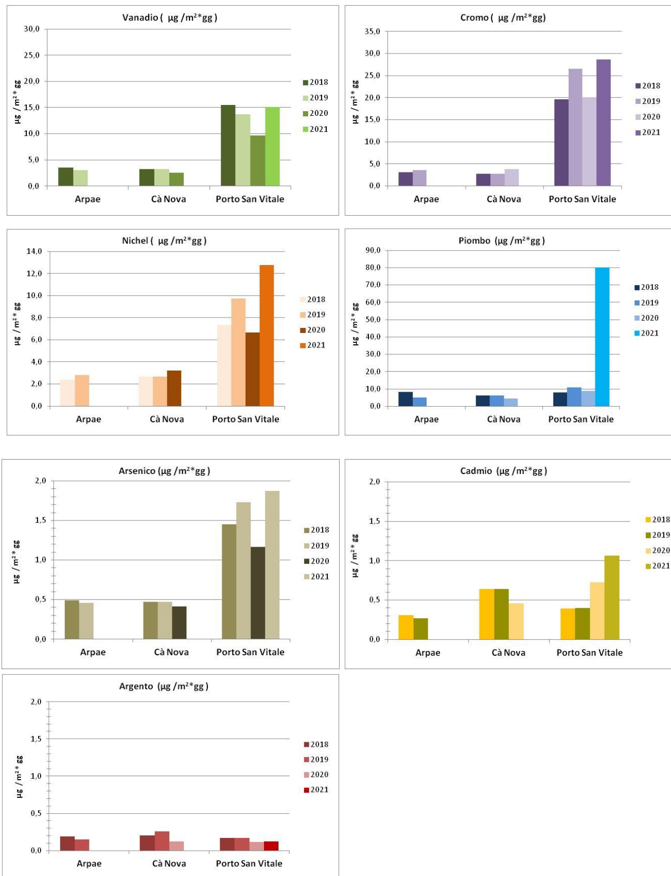
Figura 4.45: Andamento medie annuali dei metalli nelle deposizioni: 2018-2021
