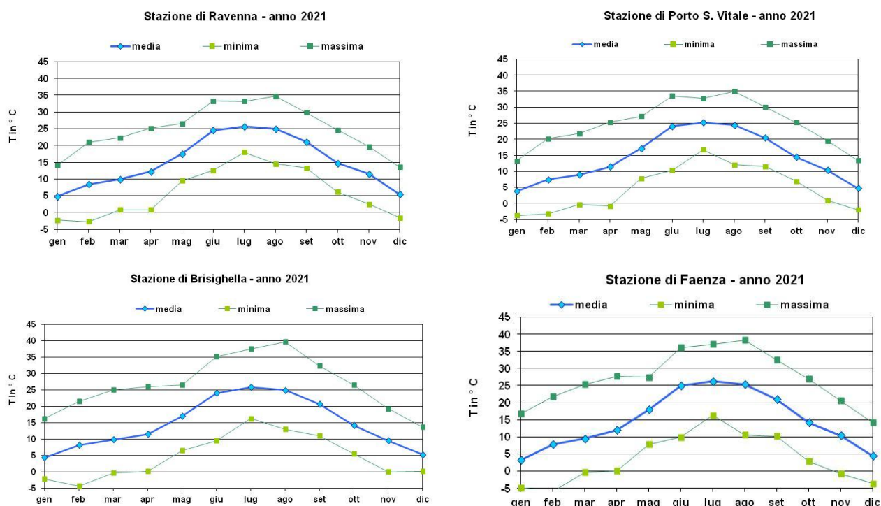
Figura 3.2d: Medie, minimi e massimi mensili delle temperature nelle stazioni di Ravenna e provincia Anno 2021
