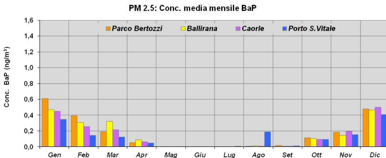
Figura 4.28 – Andamento temporale delle concentrazioni medie mensili di BaP sul PM2,5 Anno 2021
