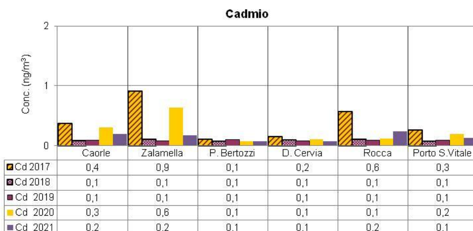
Figura 4.36 – Andamento medie annuali di alcuni metalli nel particolato PM10 – Anni 2017 ÷ 2021
