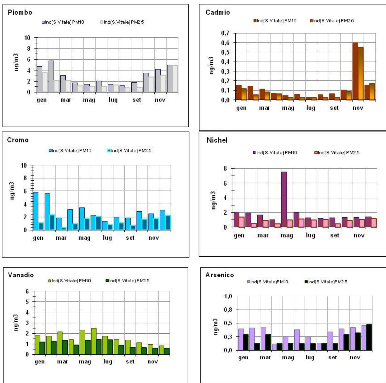
Figura 4.35 – Medie mensili di alcuni metalli nel particolato PM10 e PM2.5 – Anno 2021
