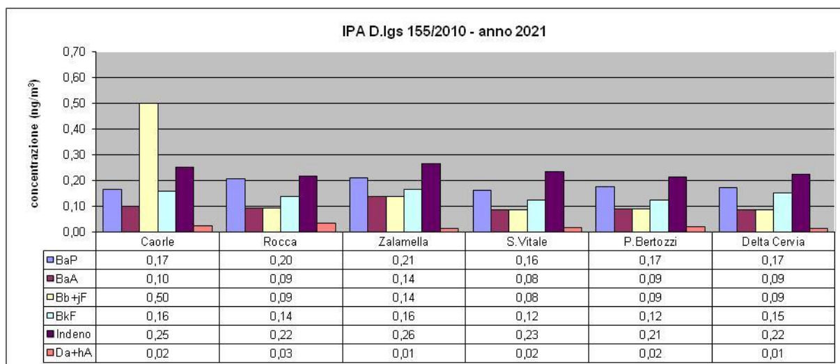
Figura 4.27 – Media annuale sul particolato PM10 (2021) degli IPA indicati dal D.lgs. 155/2010 - postazioni della rete di controllo della qualità dell'aria
