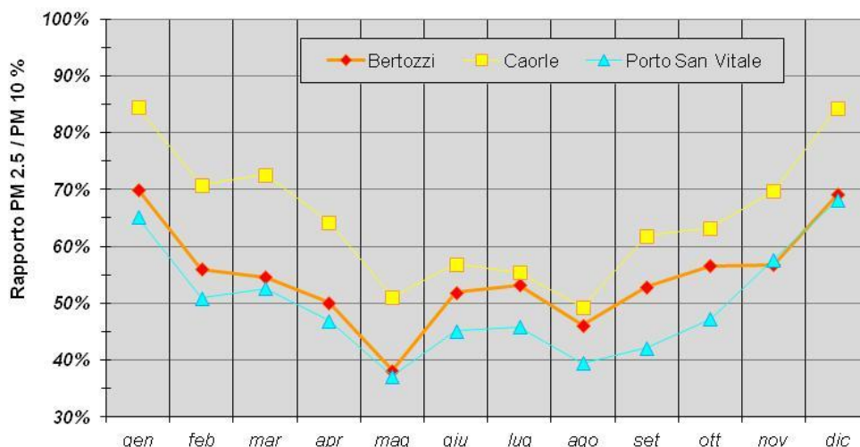
Figura 4.24 Rapporto PM2.5/PM10: medie mensili 2021 (quale % del PM10 è PM2.5)
