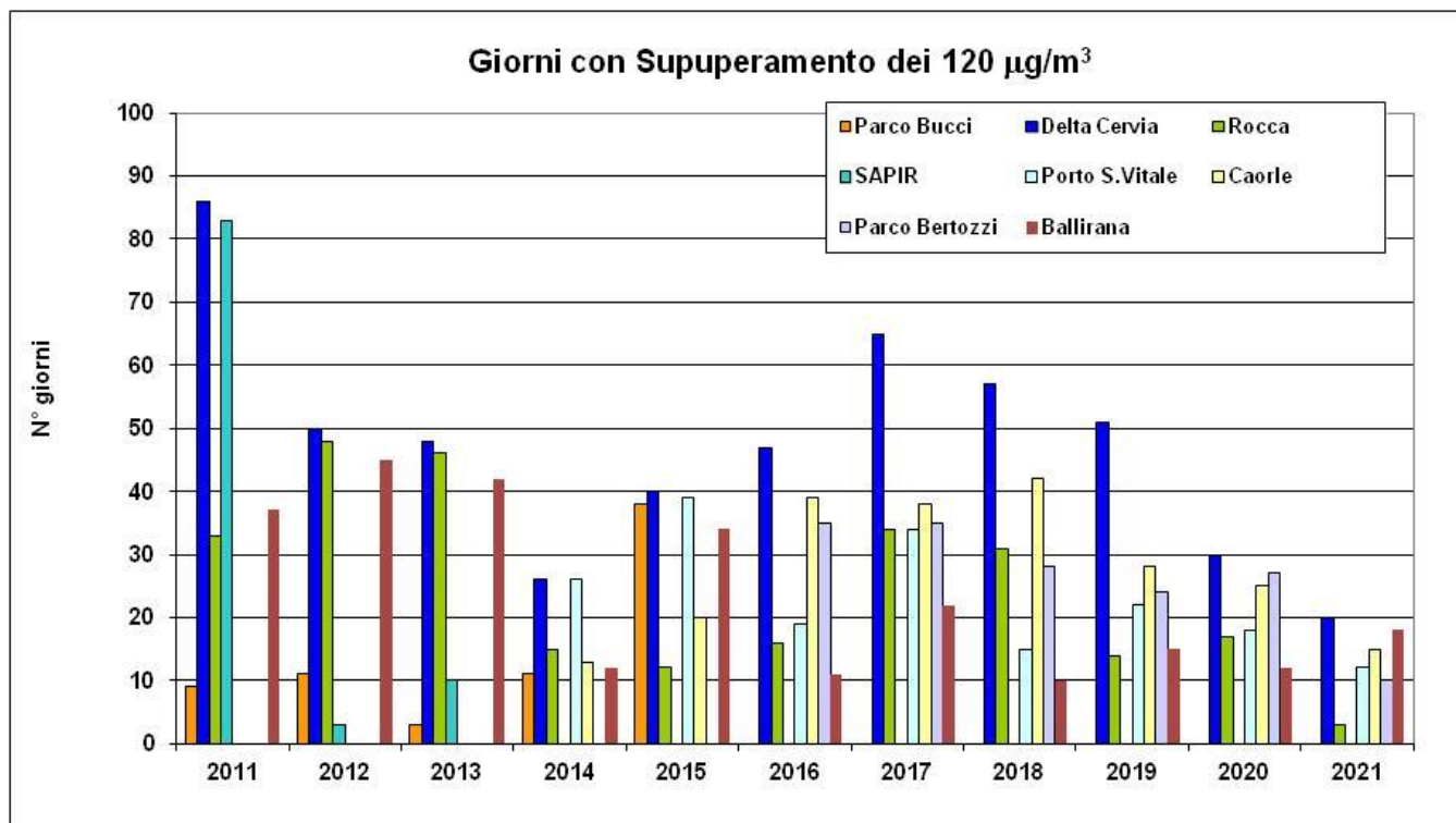
Figura 4.11 Giorni con superamento dei 120 \mu\text{g}/\text{m}^3 - periodo 2011 - 2021
