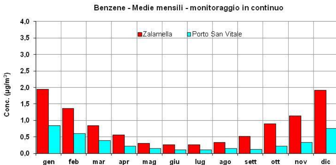
Figura 4.13 - Concentrazioni medie mensili: Zalamella e Porto San Vitale - monitoraggio continuo - Anno 2021
