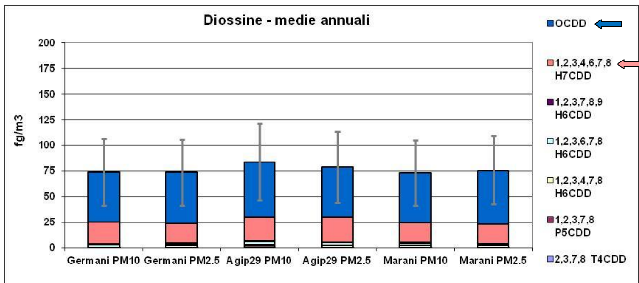
Figura 4.39 – concentrazioni medie annuali di diossine nel particolato – Anno 2021
