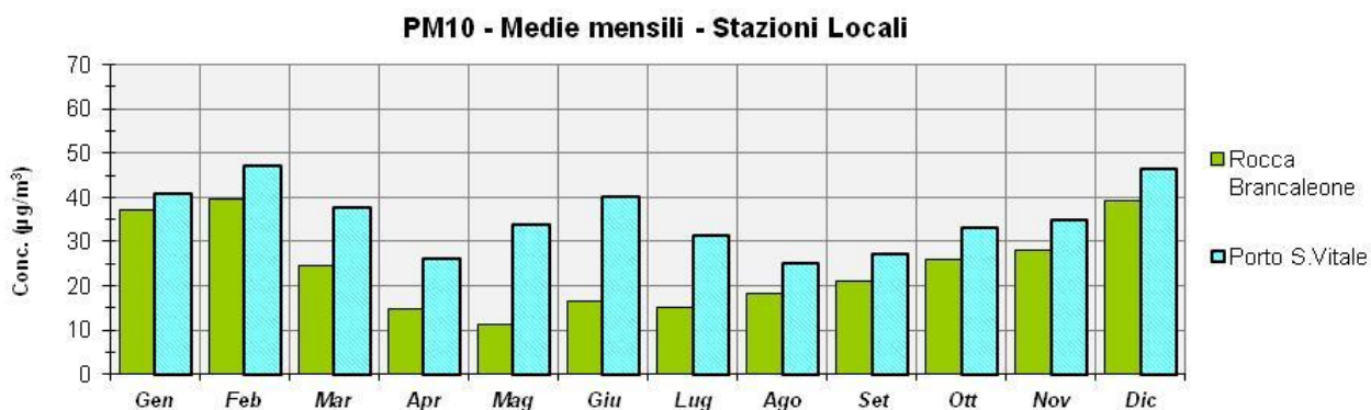
Figura 4.21 – PM10 medie mensili Area Industriale/Portuale – Stazioni Locali Industriali – anno 2021
