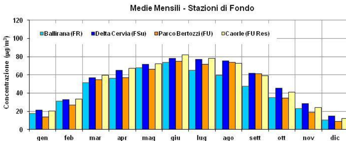
Figura 4.8 Concentrazioni medie mensili Stazioni di Fondo – anno 2021
