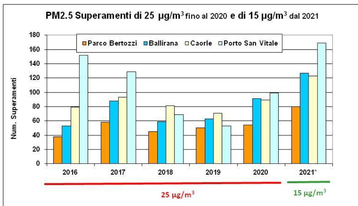
Figura 4.23 – PM2.5: medie annuali e superamenti della media giornaliera di 25 µg/m 3 nell'intervallo 2016 - 2021
