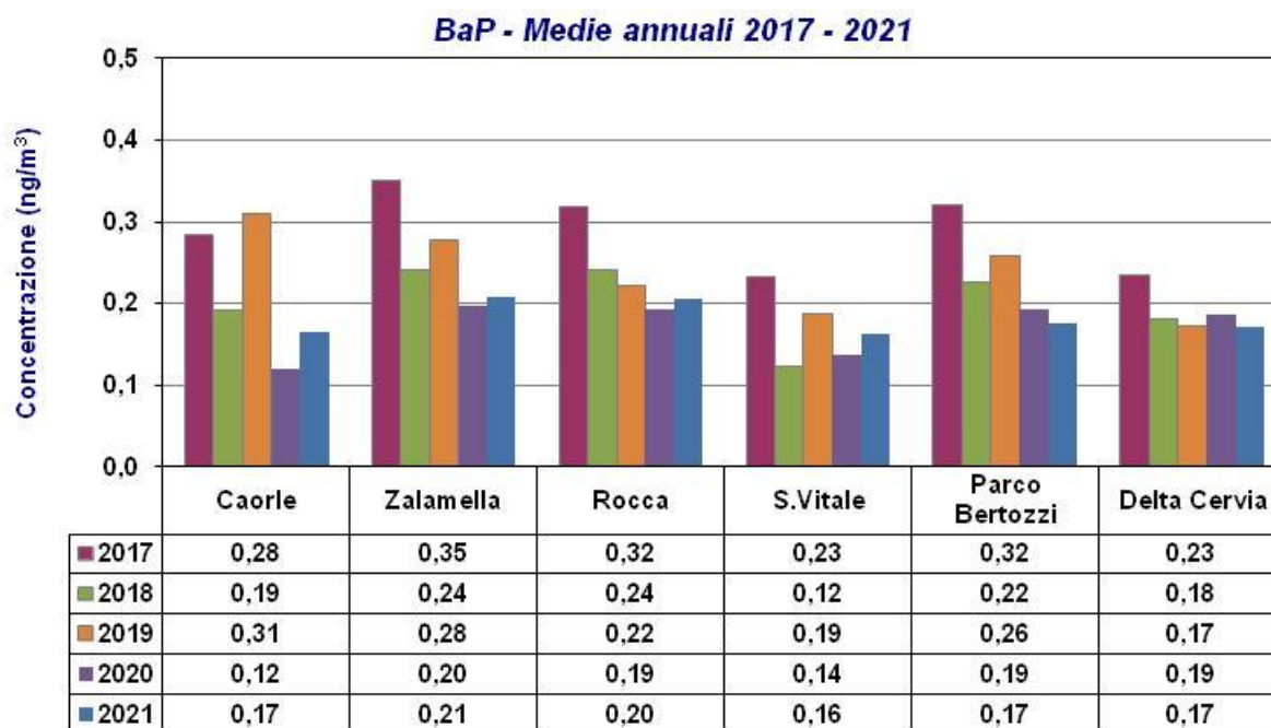
Figura 4.25 – Concentrazioni medie annuali BaP – anni 2017 – 2021
