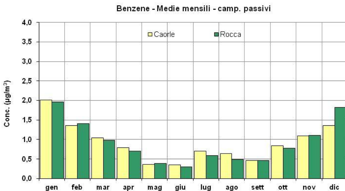
Figura 4.14 - Concentrazioni medie mensili: Caorle, Rocca - campionatori passivi - Anno 2021
