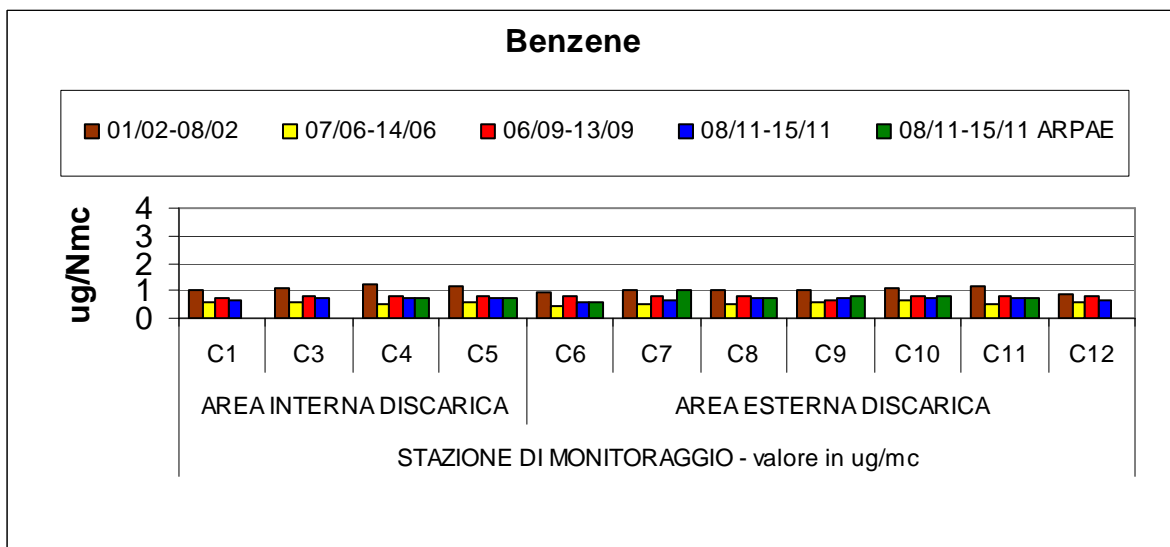
Grafico n. 4 – Andamento Benzene, anno 2021
