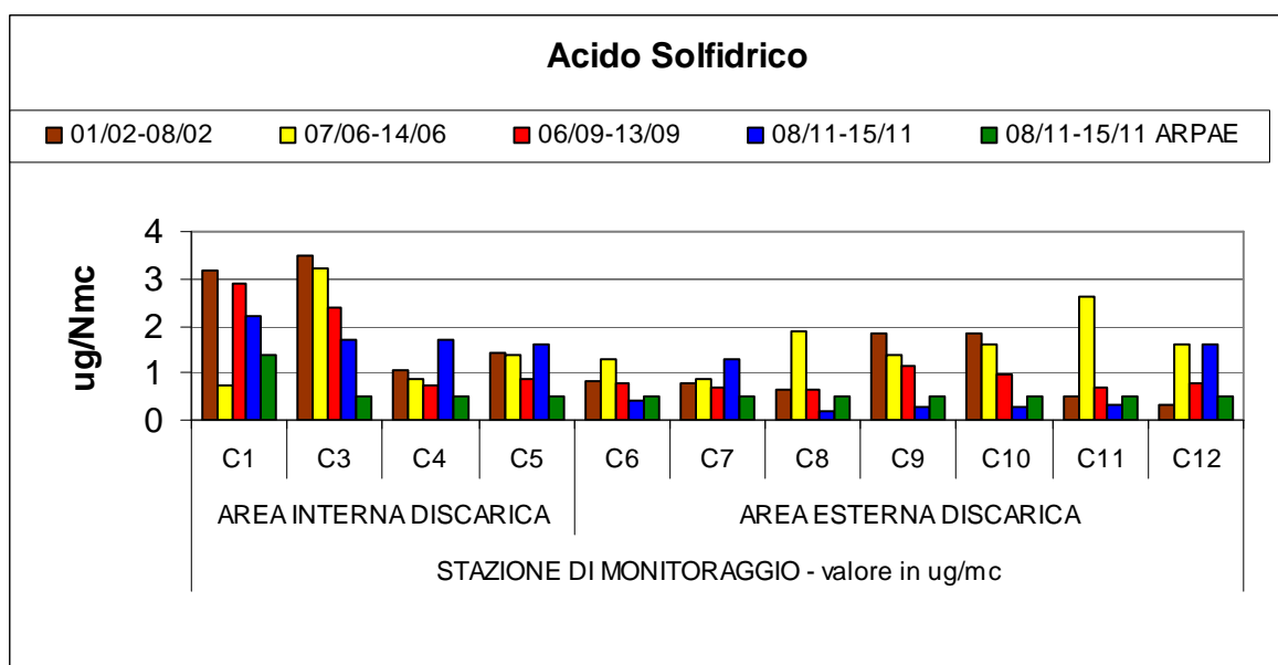
Grafico. n 7 – Andamento Acido Solfidrico, anno 2021
