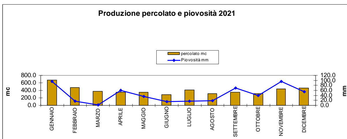
Grafico n. 2 – Andamento della produzione di percolato e piovosità nell’anno 2021
