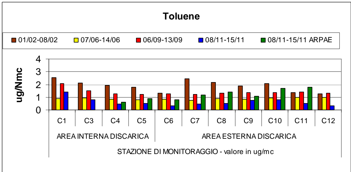
Grafico n. 5 – Andamento Toluene, anno 2021
