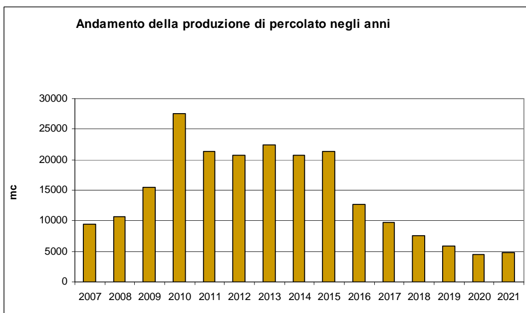
Grafico n. 3 – Andamento della produzione di percolato negli anni
