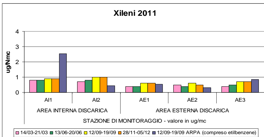
Grafico n. 4 – Andamento Xileni, anno 2011
