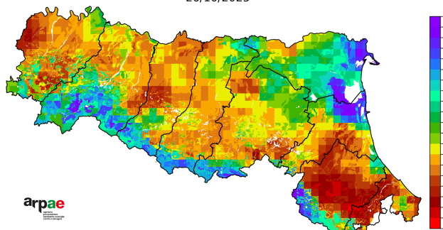
Acqua disponibile nel suolo rispetto al clima 2001-2020 (percentile) 26/10/2025
