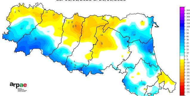
Anomalia percentuale delle precipitazioni da inizio anno (%) dal 01/01/2025 al 26/10/2025
