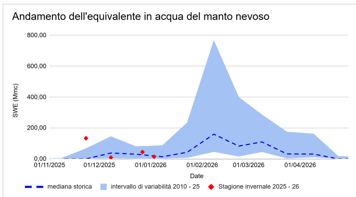
Figura 3 - Il grafico mostra l'andamento nel tempo dei valori di Snow Water Equivalent (SWE) in Mmc (punti rossi), confrontato con la mediana dell'archivio storico di SWE 2010-2025 (linea tratteggiata) e l'intervallo di variabilità (fascia azzurra), delimitato in alto dal 75° e in basso dal 25° percentile. I dati di SWE sono mediati sul territorio di competenza idrografica della Regione Emilia-Romagna.
