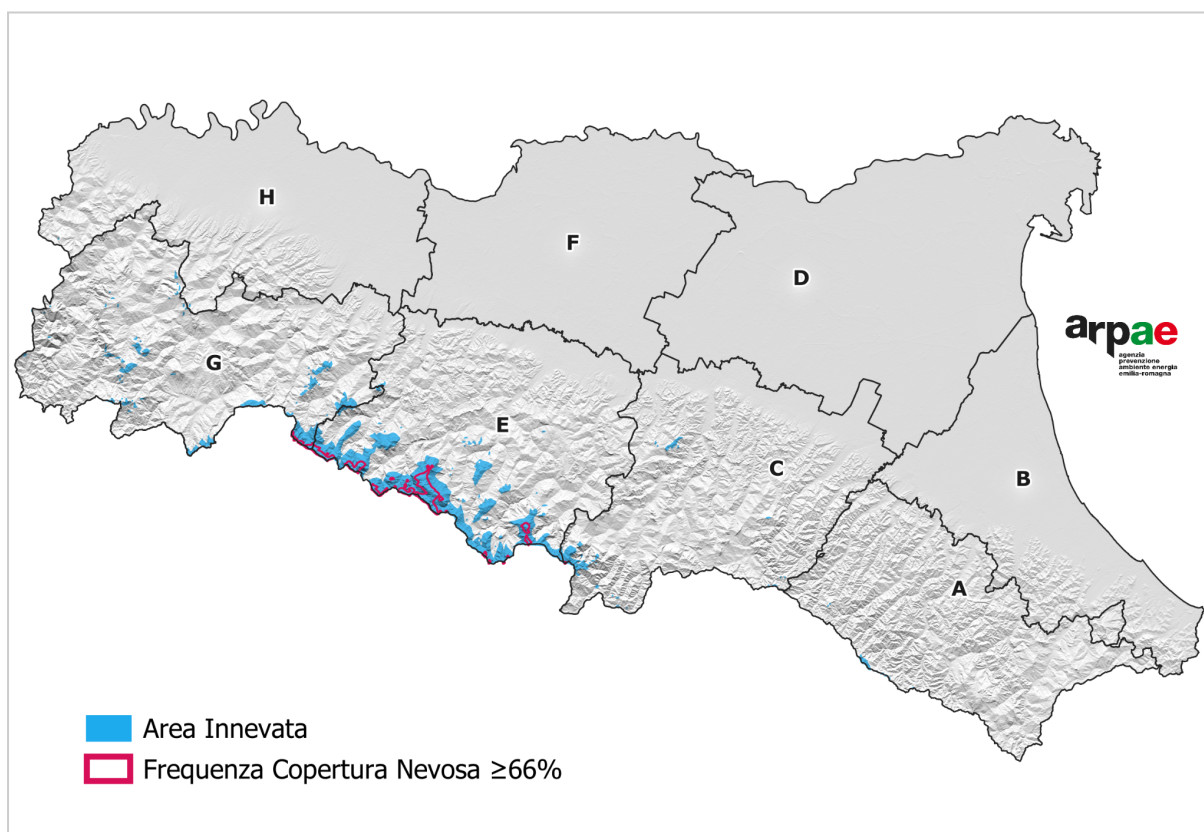
Figura 5 - Mappa dell'innevamento da dati satellitari e modellistici sulle macroaree omogenee dal punto di vista climatologico e idrologico della Regione Emilia-Romagna. La presenza di copertura nevosa viene mostrata in azzurro, mentre i contorni di colore rosso rappresentano le zone in cui, nell'intervallo di riferimento 2000 - 2025, è stata rilevata la presenza di neve con frequenza maggiore o uguale al 66% nella metà del mese in cui ricade l'immagine satellitare del presente bollettino.
