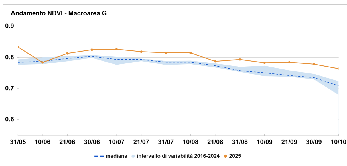
Figura 5 - Macroarea G: il grafico mostra l'andamento della mediana dell'indice NDVI dell'anno in corso (linea arancione) confrontato con la mediana del periodo 2016-2024 (linea tratteggiata) e l'intervallo di variabilità (fascia azzurra), delimitato in alto dal 75° e in basso dal 25° percentile.
