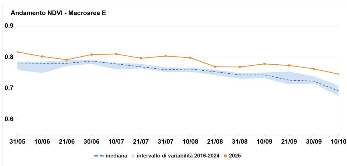
Figura 4 - Macroarea E: il grafico mostra l'andamento della mediana dell'indice NDVI dell'anno in corso (linea arancione) confrontato con la mediana del periodo 2016-2024 (linea tratteggiata) e l'intervallo di variabilità (fascia azzurra), delimitato in alto dal 75° e in basso dal 25° percentile.
