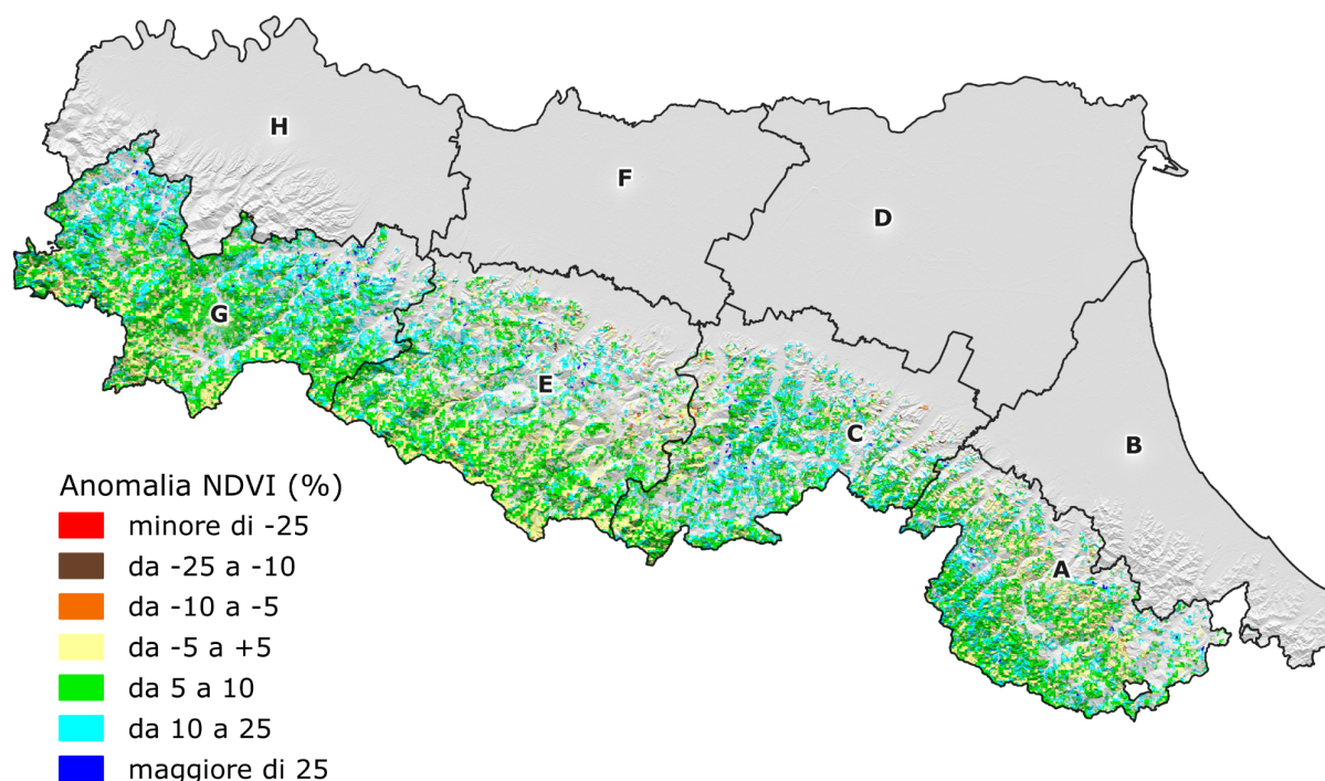
Figura 1 - Anomalia di NDVI sulle macroaree a elevata copertura forestale rispetto alla serie 2016-2024
