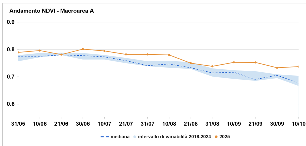
Figura 2 - Macroarea A: il grafico mostra l'andamento della mediana dell'indice NDVI dell'anno in corso (linea arancione) confrontato con la mediana del periodo 2016-2024 (linea tratteggiata) e l'intervallo di variabilità (fascia azzurra), delimitato in alto dal 75° e in basso dal 25° percentile.
