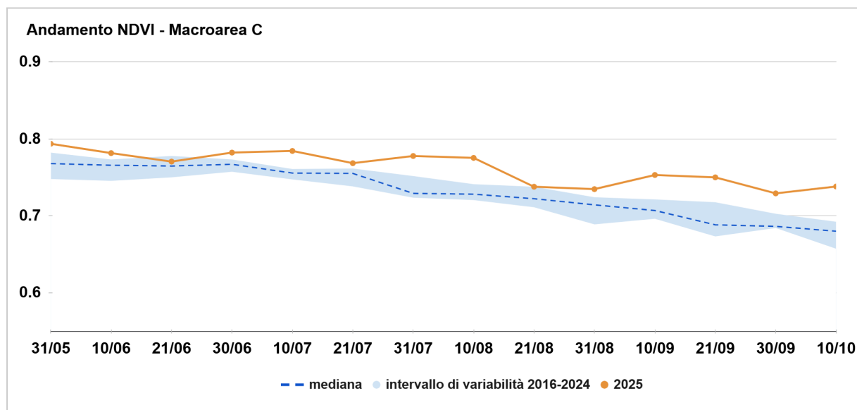
Figura 3 - Macroarea C: il grafico mostra l'andamento della mediana dell'indice NDVI dell'anno in corso (linea arancione) confrontato con la mediana del periodo 2016-2024 (linea tratteggiata) e l'intervallo di variabilità (fascia azzurra), delimitato in alto dal 75° e in basso dal 25° percentile.
